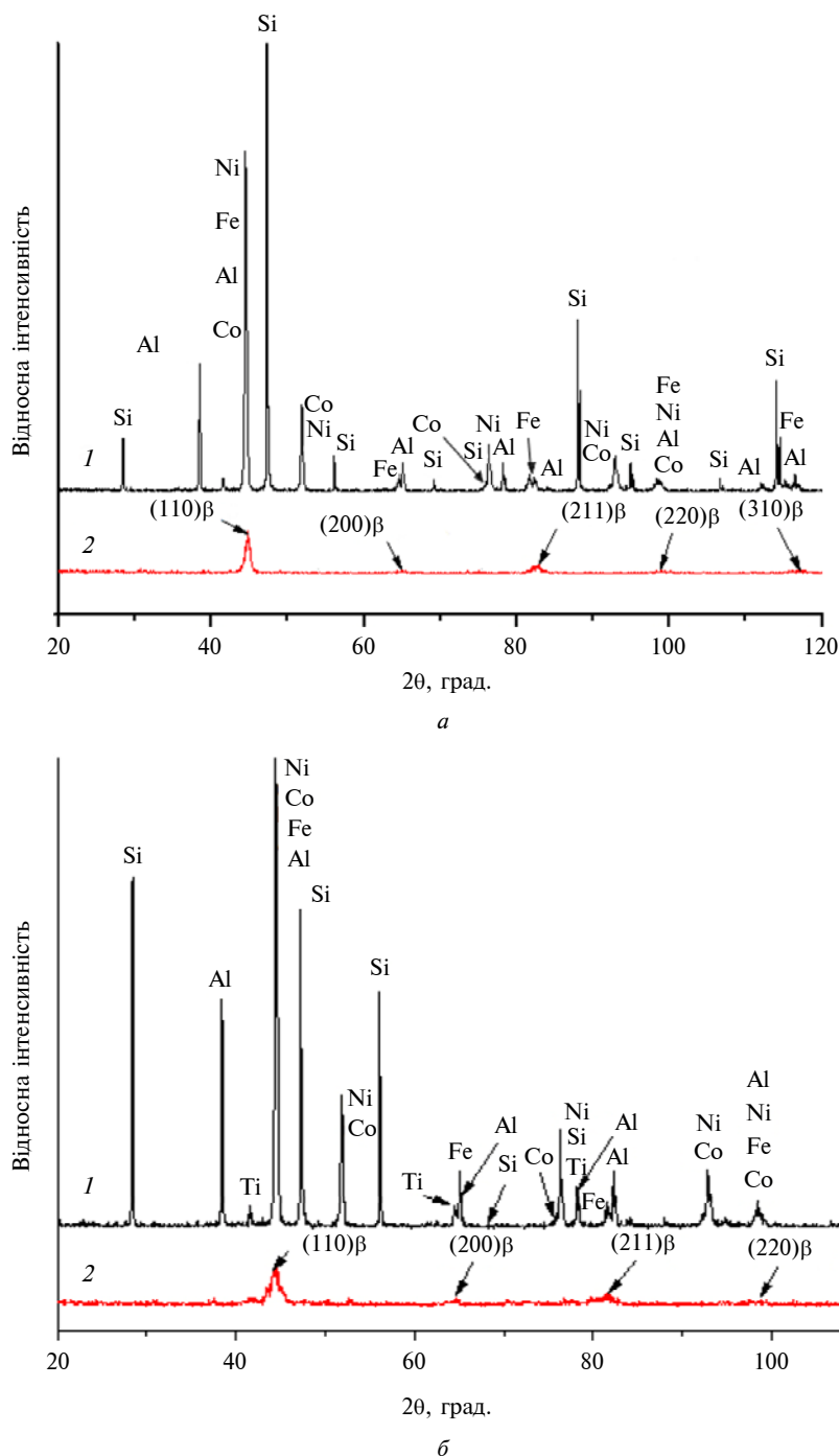
Рис. 2. Дифракційні спектри вихідної суміші порошків (1) та AlSiNiCoFeCr (а) і AlSiNiCoFeCrTi (б) високоентропійних покриттів (2), отриманих електронно-променевим наплавленням
