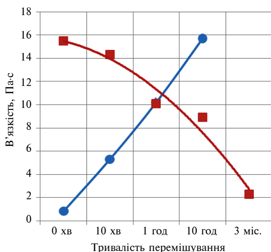
Рис. 6. Залежність ефективної в'язкості глинисто-карбонатної суспензії від тривалості перемішування: ● — перемішування, ■ — стан спокою
