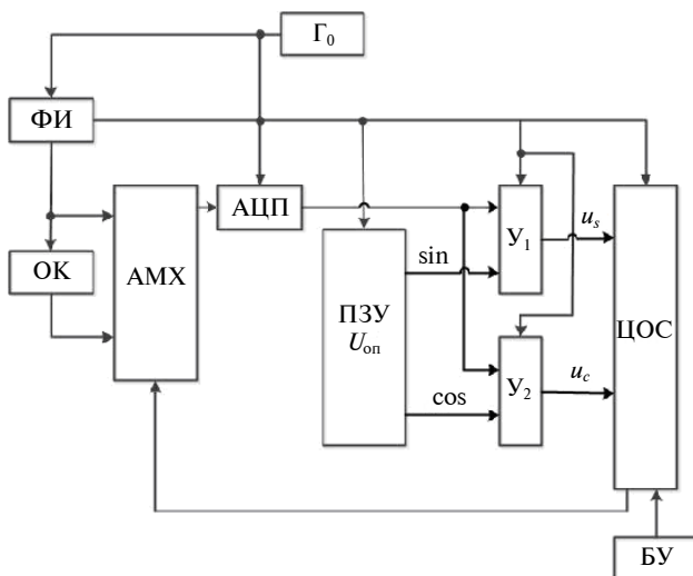
Рис. 2. Структурная схема измерителя фазового сдвига: ФИ – формирователь радиоимпульсов; АМХ – аналоговый мультиплексор АЦП; ОК – объект контроля; \Gamma_0 – высокостабильный генератор сигналов частоты дискретизации; ПЗУ – постоянное запоминающее устройство; Y_1 , Y_2 – умножители цифровых сигналов; ЦОС – блок цифровой обработки сигналов; БУ – блок управления
