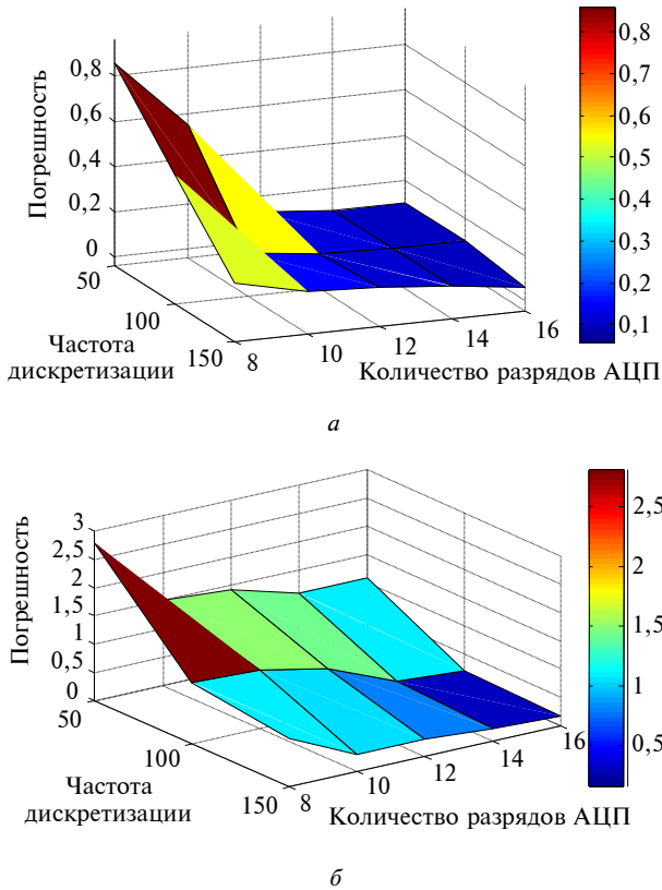
Рис. 1. Зависимость погрешности измерения ФС от параметров АЦП для \varphi = 90^\circ : а – f = 0,5 МГц, б – f = 2,5 МГц
