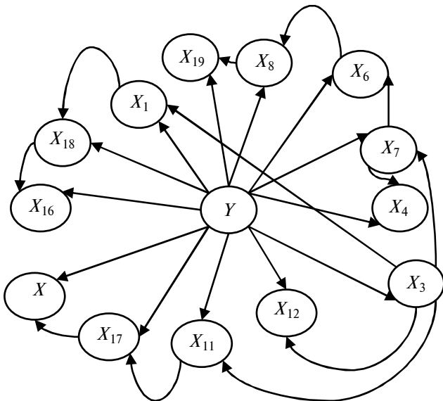
Рис. 5. Доповнена деревом байєсівська мережа для набору даних German Bank Accepts
