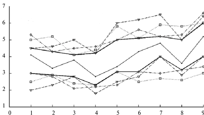
Рис. 4. Графічні результати обчислення інтервального прогнозу узагальнювальної інтервальної нечіткої моделі типу 2: —■— експериментальне значення; —▽— інтервальний прогноз 1-ї часткової моделі; - - - □ - - - інтервальний прогноз 2-ї часткової моделі; -◇- - - інтервальний прогноз 3-ї часткової моделі; ——— інтервальний прогноз узагальнювальної моделі
