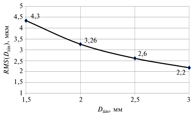
Рис. 3. Графік залежності RMS(D_{\text{зін}}) при дифракційно-обмеженій якості зображення точки на сітківці ока
