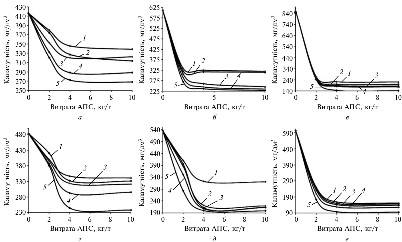
Рис. 1. Залежність каламутності підсіткової води від витрат АПС за використання макулатури марки МС-5Б-2 за ступеня млива: 35 °ШР (а), 50 °ШР (б), 55 °ШР (в); та макулатури марки МС-8В-3 за ступеня млива: 50 °ШР (г), 55 °ШР (д), 60 °ШР (е); 1 – Luresin KS; 2 – Eka WS 325; 3 – Kumene 25X-Cel; 4 – Fennostrength PA21; 5 – Ультрарез 200
