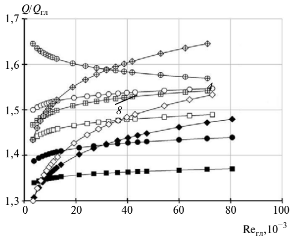
Рис. 2. Залежності Q/Q_{г\text{л}} = f(Re_{г\text{л}}) при \Delta P/\Delta P_{г\text{л}} = \text{idem} та \sigma_1 = 1,105 : 1, 2, 3 – \sigma_2 = 0,96 для труби типу 1, типу 2, типу 3 відповідно; 4, 5, 6 – \sigma_2 = 1,184 для труби типу 1, типу 2, типу 3 відповідно; 7, 8, 9 – \sigma_2 = 1,46 для труби типу 1, типу 2, типу 3 відповідно
