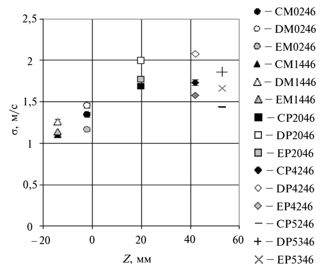
Рис. 3. Зміна с.к.в. трансверсальної швидкості в досліджуваній зоні ЕКВС за різних видів зовнішнього збурення
